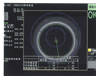
画像処理
