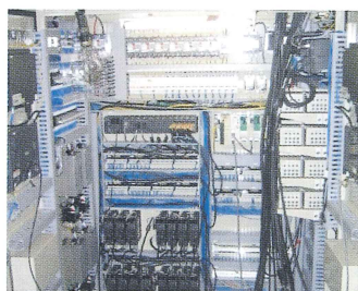
制御盤製作
